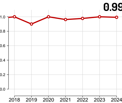
Cociente entre los créditos cursados aptos y los créditos cursados matriculados de los alumnos de una cohorte de egreso
