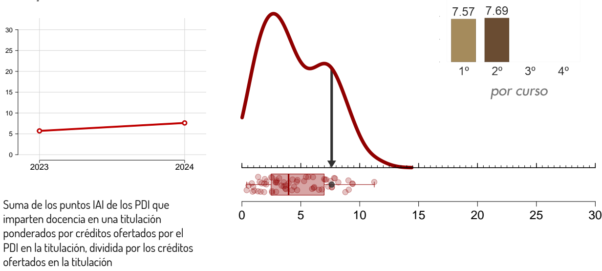
IAI_ponderado 7.619
